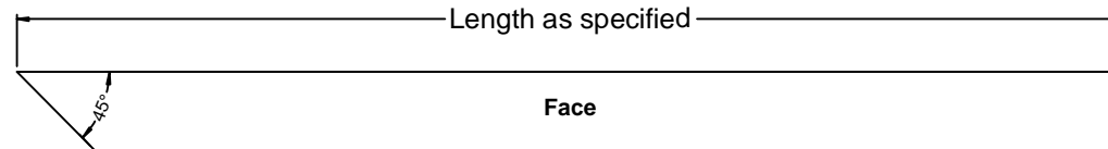
MOE/LH Mitred One End - Left Hand
